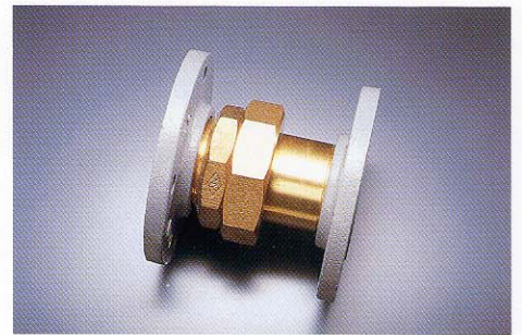
伸縮式ユニオン継手(両フランジ式) ●寸法/75、100mm
