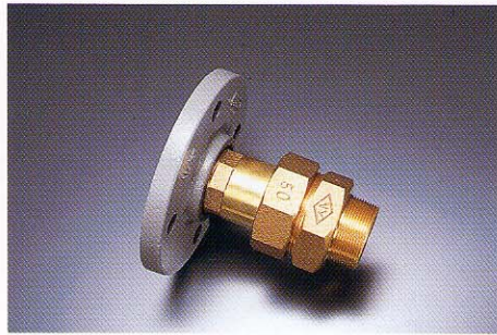
伸縮式ユニオン継手(片フランジ式) ●寸法/50、75、100mm
