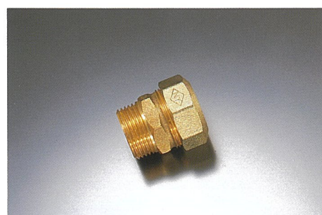
外ネジ(塩ビ管用ソケット) ●寸法/13~50mm
