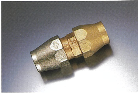
PVソケット (ポリ管とビニル管を接続) ●寸法/13~50mm ※異径はP13×V16、P20×V13、P20×V16、 P50×V40、P50×V25mm
