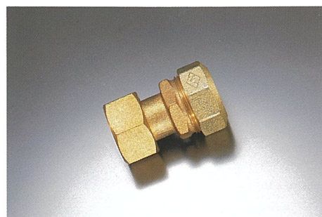
メーター用ソケット ●寸法/13~25mm
