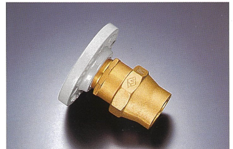
合フランジ付Pソケット(コア付) ●寸法/50mm
