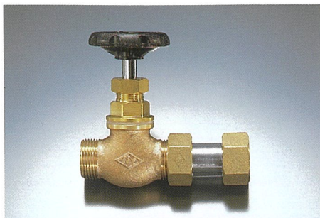
伸縮式直結メーター止水栓(本管側用) ●寸法/13~50mm ※本体のみ、ビニル管用、鉄管用
