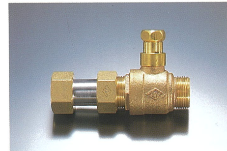
伸縮式ボール止水栓(盗水防止型) ●寸法/13~25mm ※本体のみ、ビニル管用、鉄管用
