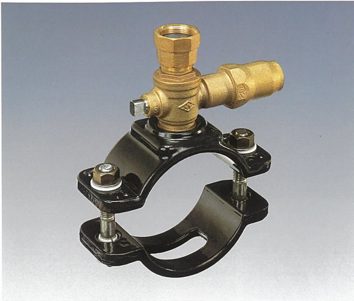
NY式サドル分水栓(伸縮型)
