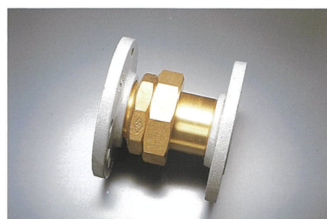
伸縮式ユニオン継手(両フランジ式) ●寸法/75、100mm
