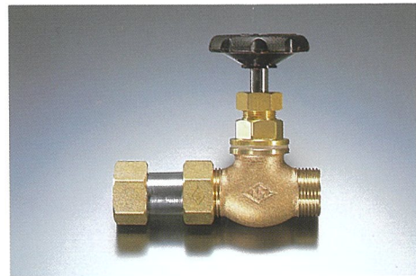
伸縮式直結メーター止水栓(家庭側用) ●寸法/13~50mm ※本体のみ、ビニル管用、鉄管用
